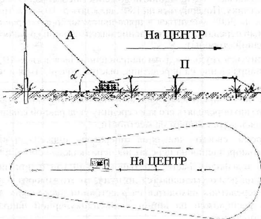
Рис.8.4 Диаграмма направленности антенны «наклонный луч»
