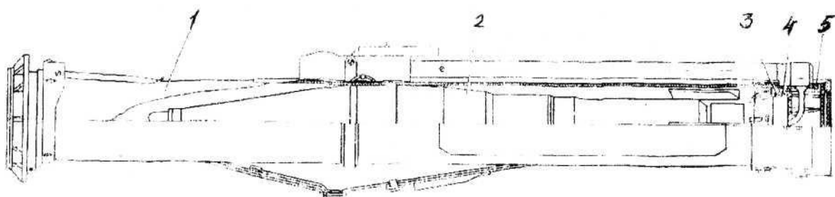
Рис. 4.25 Устройство РПГ-26:
