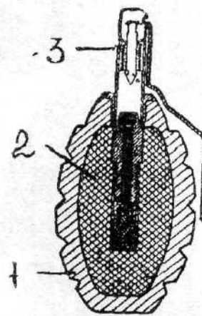
Рис. 4.37 Устройство Ф-1: 1 корпус; 2. разрывной заряд; 3 запал.
