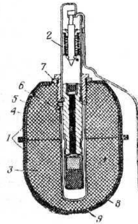
Рис. 4.35 Устройство РГД-5:
