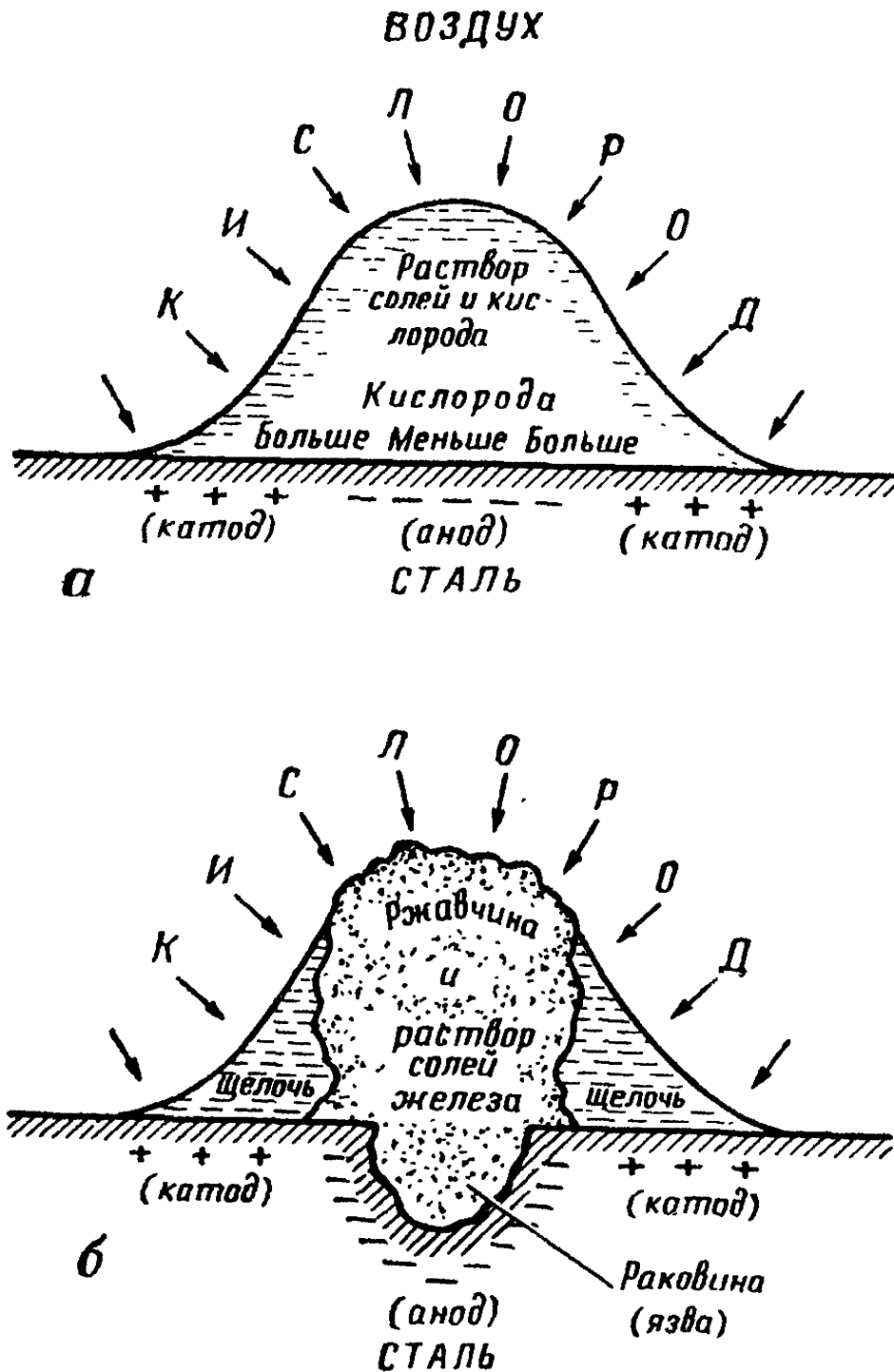
Рис. 2. Схема коррозии стали под каплей электролита: а -- начальная стадия коррозии; б -- результат коррозии
