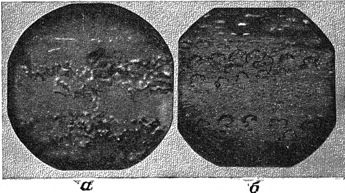
Рис. 6. Коррозия не вычищенного после стрельбы нехромированного ствола винтовки:
