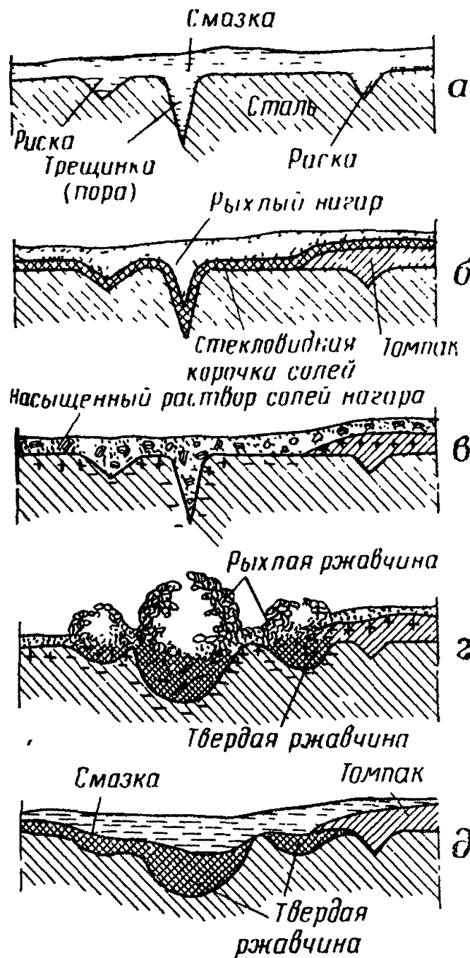
Рис. 4. Схема коррозии каналов нехромированных стволов стрелкового оружия:
