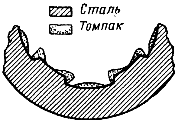
Рис. 3. Схема расположения томпакизации в каналах стволов стрелкового оружия
