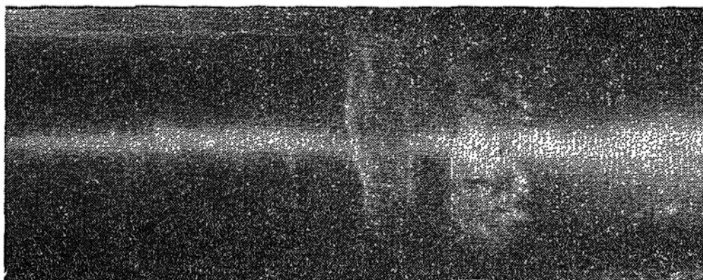
Рис. 12. Коррозия нехромированного штока накатника артиллерийского оружия под воротником (матовая шейка с мелкими раковинами)
