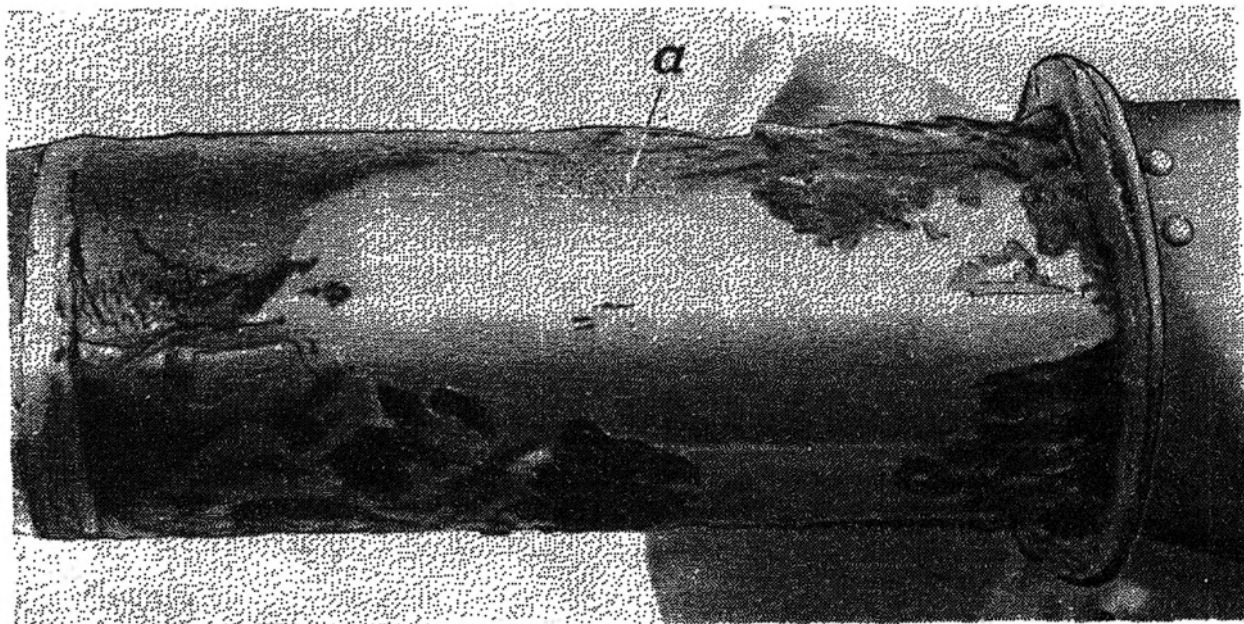
Рис. 13. Сползание пушечной смазки с цилиндрической полированной части ствола пушки:
