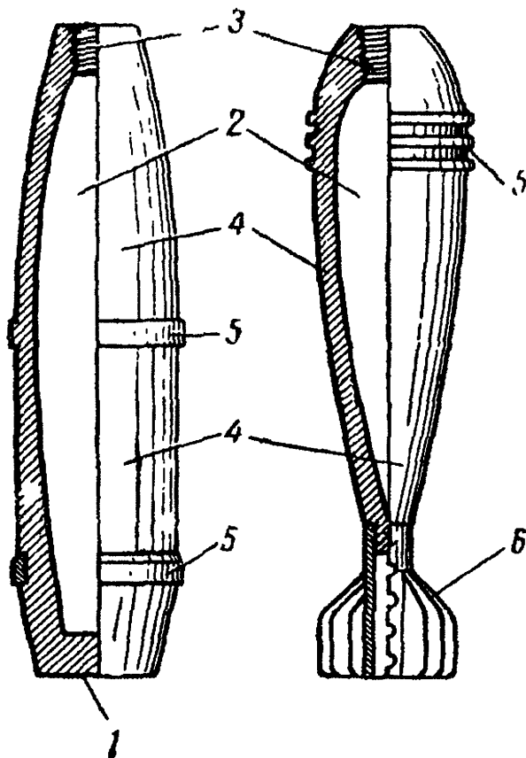
Рис. 14. Схема защиты снаряда и мины от коррозии:
