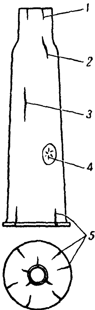
Рис. 15. Расположение трещин на латунных гильзах для орудийных выстрелов:
